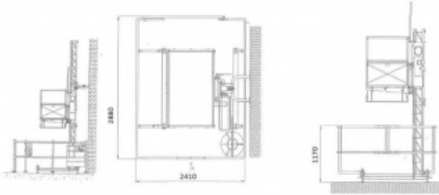
Engagement standard pour monte-charge 500 kg
