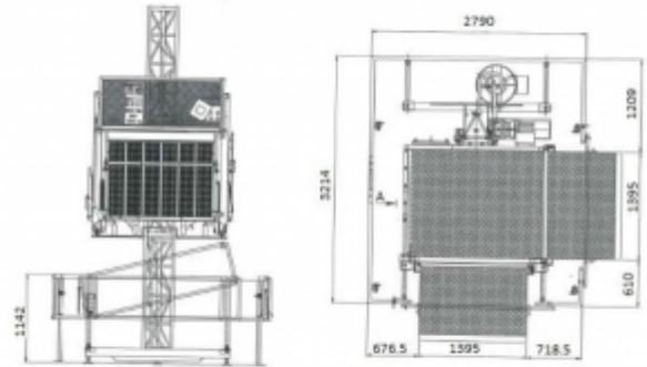
Engagement standard pour monte-charge 800 kg et monte-charge avec accompagnant 1 000 kg
